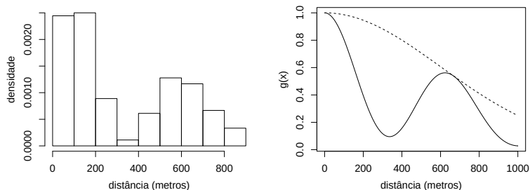
(a) Distribuição das distâncias perpendiculares observadas. (b) Função de detecção g(x) : eq. 2 (linha sólida) vs. half-normal (linha tracejada).
