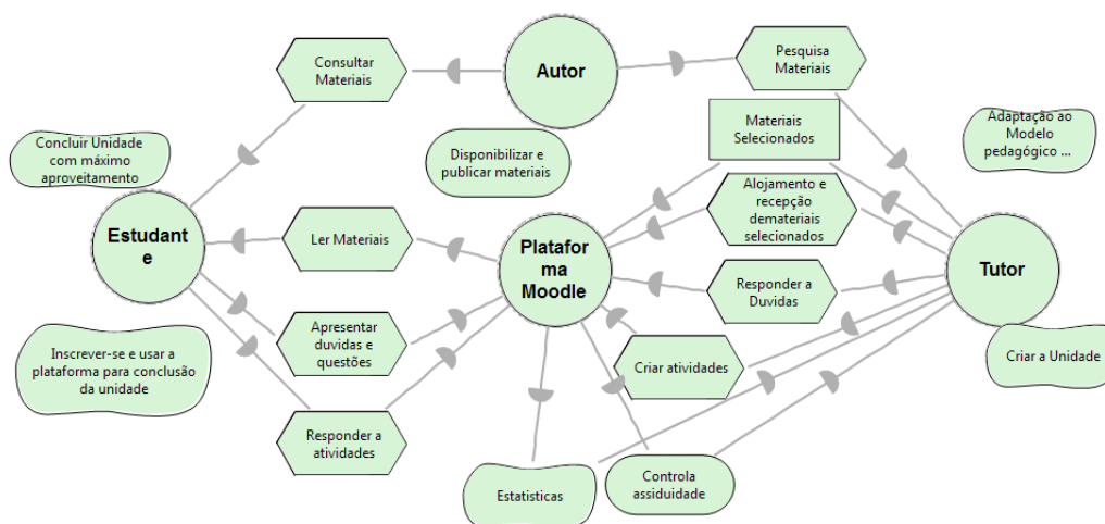
Figura 8 - Modelo de Dependência Estratégica dos Requisitos Iniciais
