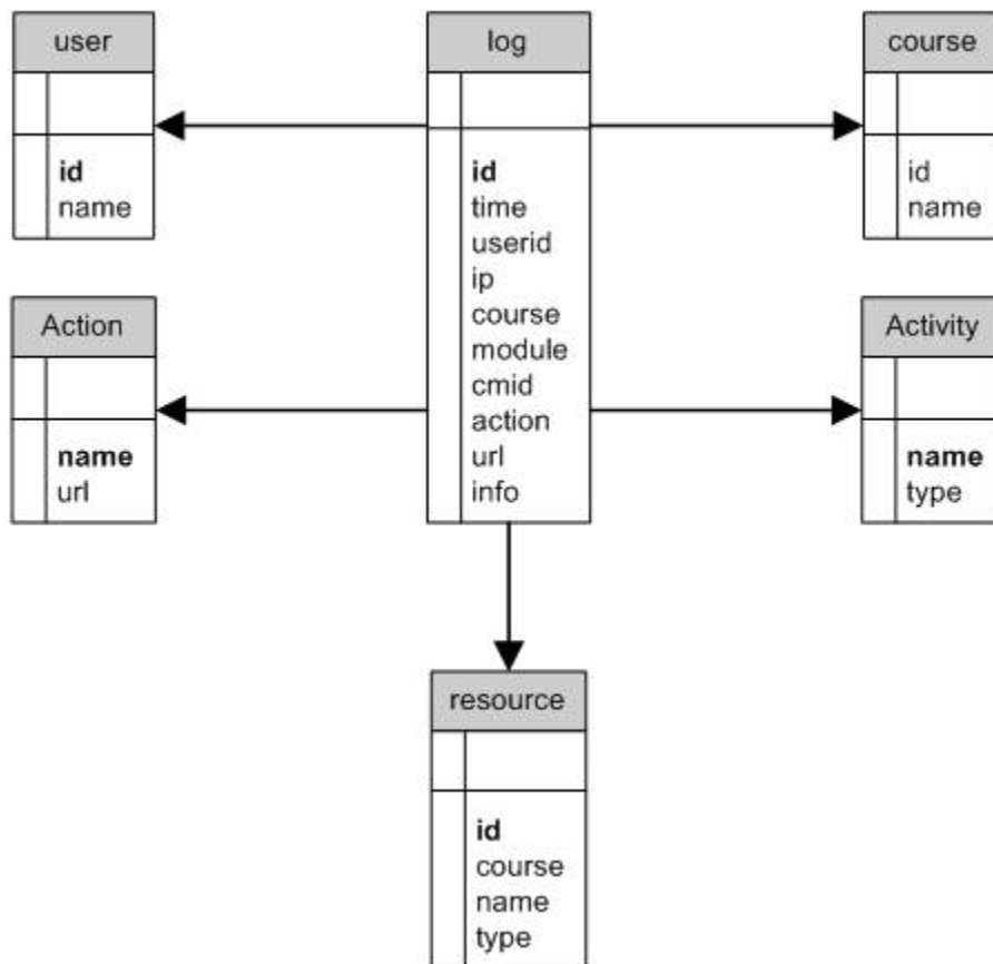
Figura 19 - Diagrama de e ligação de tabelas - Moodle
