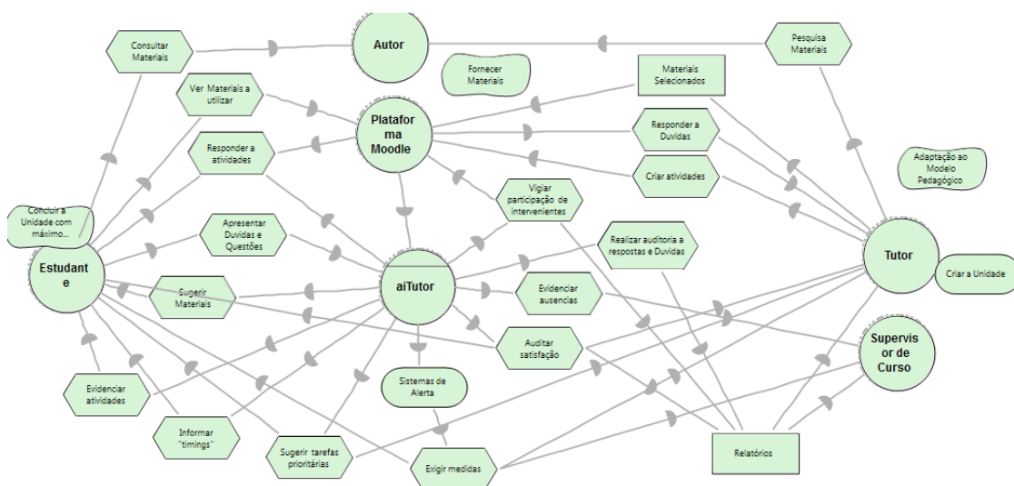
Figura 12 - Modelo de Dependência Estratégica dos Requisitos Finais
