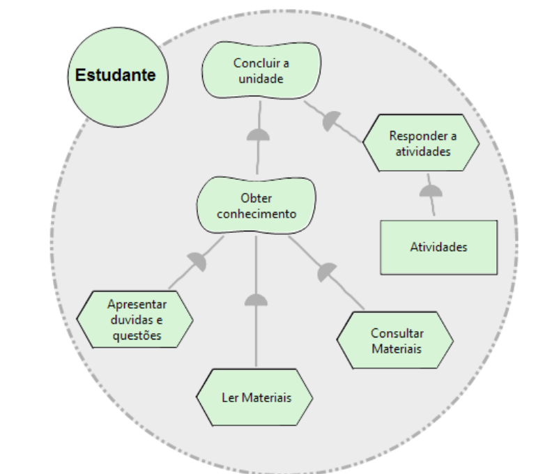
Figura 9 - Modelo I* de Razão Estratégica para o ator estudante
