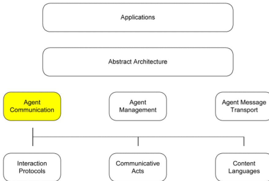
Figura 1- Estrutura FIPA
