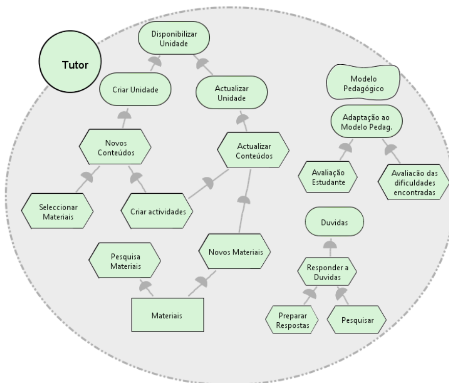
Figura 10 - Modelo I* de Razão Estratégica para o ator Tutor
