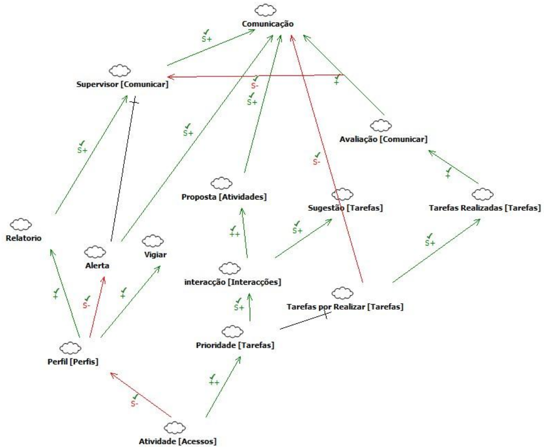
Figura 15 - Diagrama NFR baseado no estilo Integração Vertical
